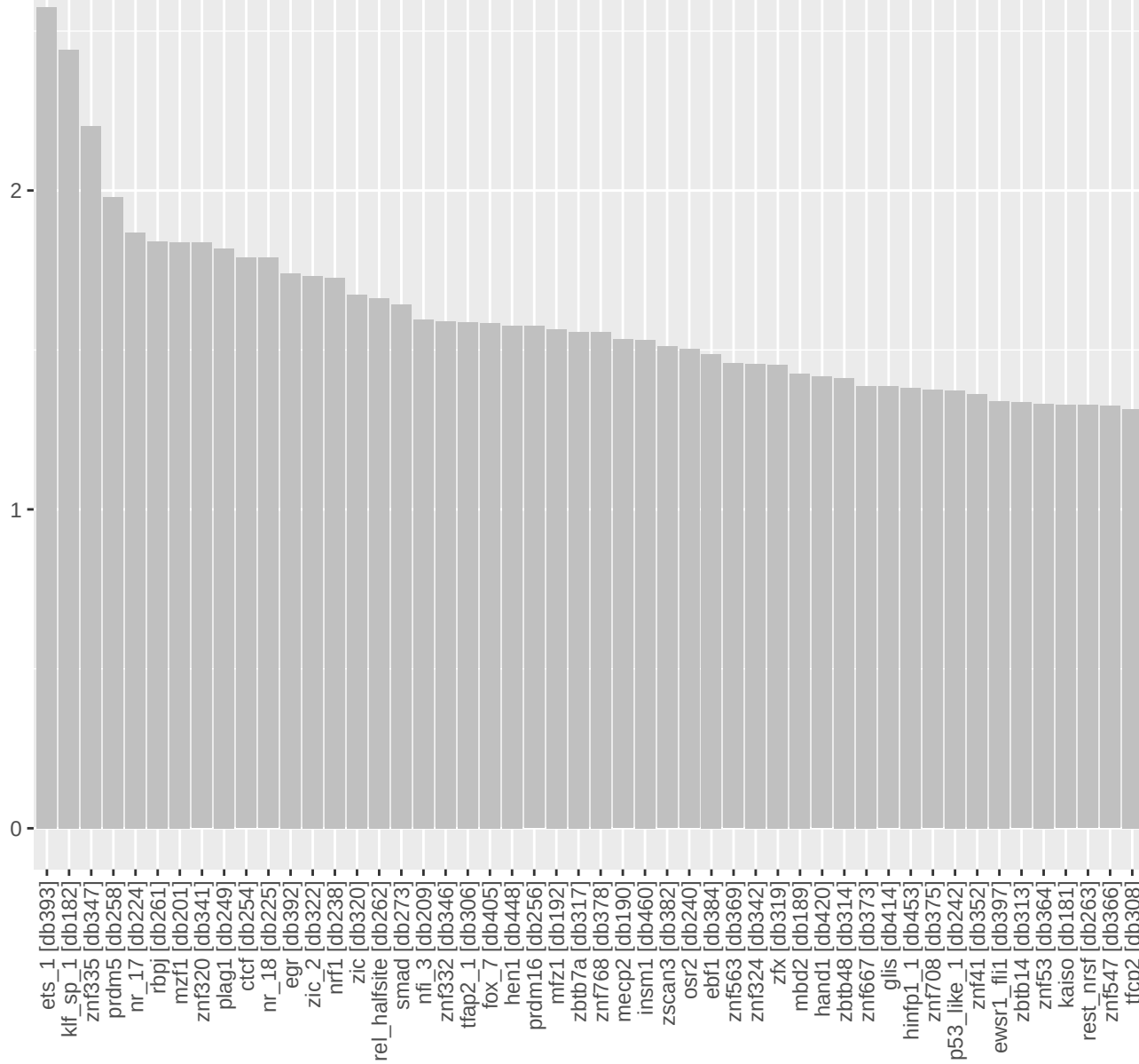
TF_motif_clusters
